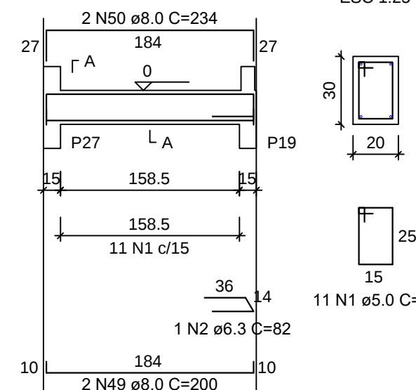
SEÇÃO A-A ESC 1:25
