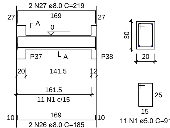
SEÇÃO A-A ESC 1:25
